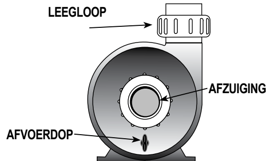
VOORAANZICHT VAN DE POMP
