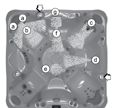
JETPOMP 2 – JETSYSTEEM 2
