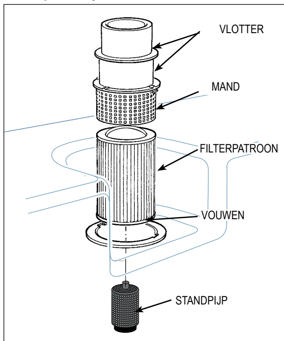
FILTERSYSTEEM
